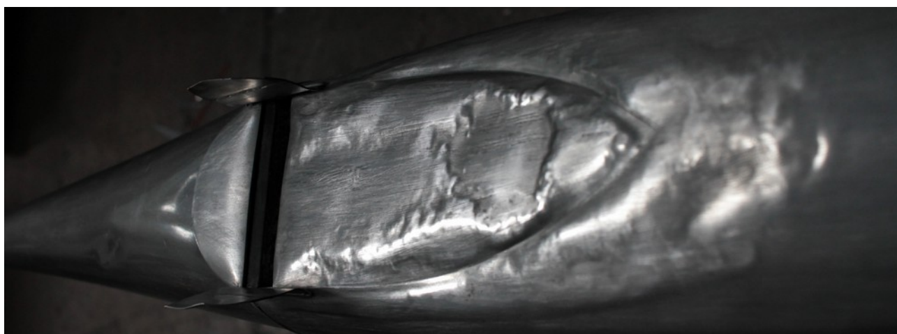
Un renfort de carton collé à l'intérieur du tuyau a provoqué d'importantes déformations du métal
