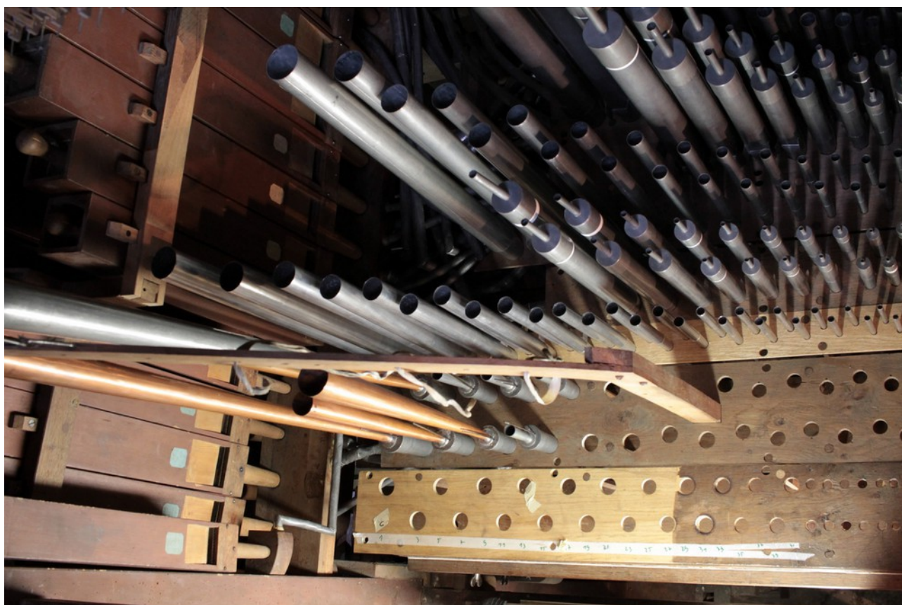
Vue de dessus du G.O. lors du remontage de la tuyauterie. La doublette neuve est en place, entre le Bourdon et la Trompette. Le faux sommier du clairon est refait partiellement, pour conserver la double perce d'origine de la dernière octave
