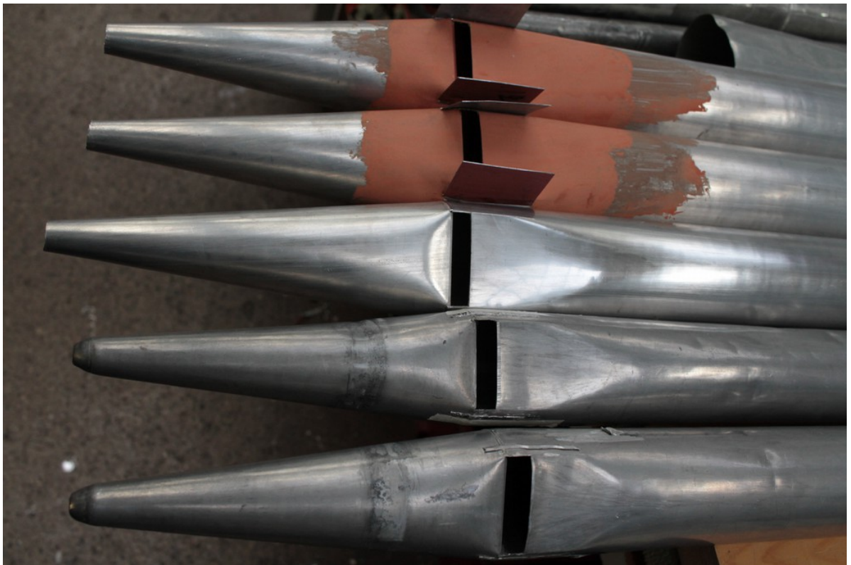
Fabrication des basses disparues du Salicional du Récit en copie de facture
